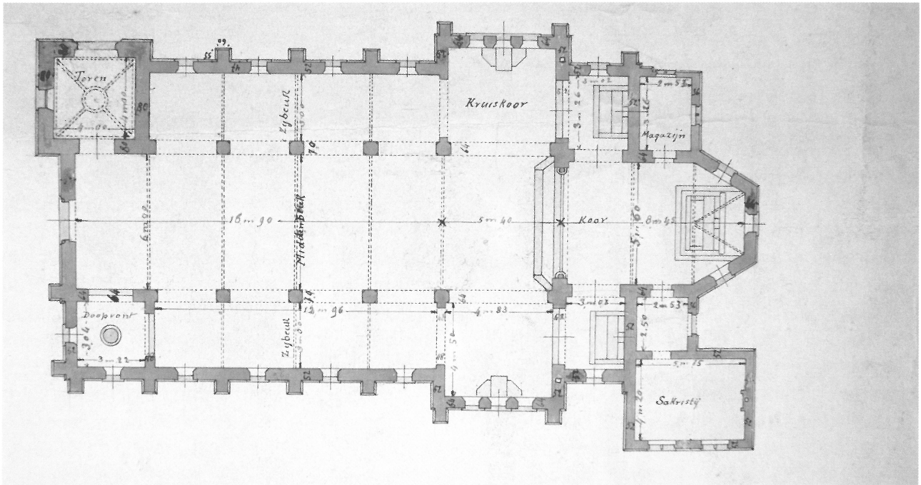
Grondplan van de kerk.
