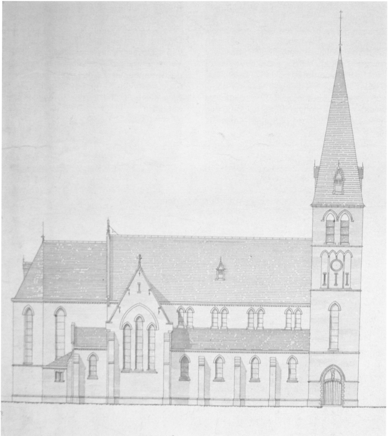
Zijaanzicht vanaf de steenweg.
